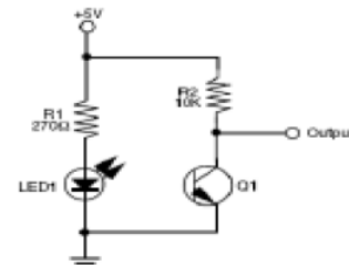
Gambar 4. Sensor Garis Sumber : (pdf Tim robotika Politeknik Elektronika Negeri Surabaya, Sensor Proximity, Surabaya, 2011, halaman 9).
