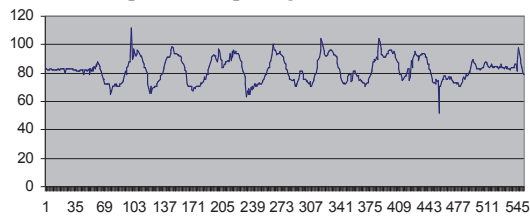
Gambar 12a Nilai ADC Accelerometer dengan K_p=5
