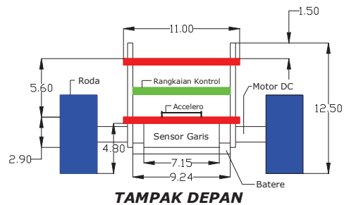
Gambar 5 Dimensi Robot Tampak Depan
