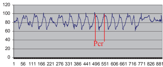
Gambar 12b Nilai ADC Accelerometer dengan K_p=10
