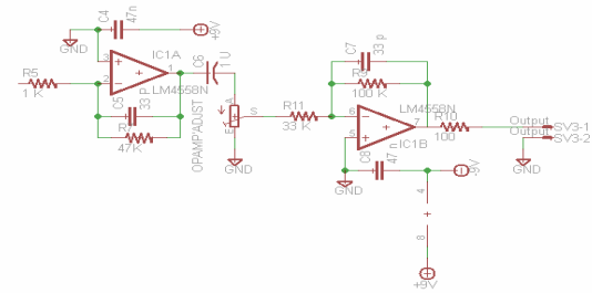
Gambar 3.2 : rangkaian amplifier
