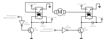
Gambar 10 rangkaian penggerak motor DC.
