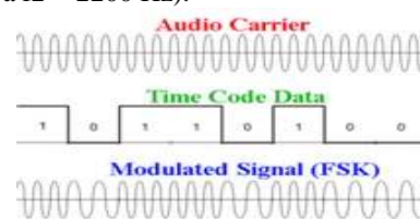
Gambar 1. Modulasi FSK
