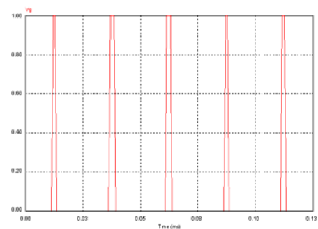
Gambar 3.7. Pulsa untuk penyulutan Mosfet Boost Converter.
