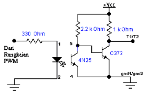
Gambar 4.2 Rangkaian Optocoupler
