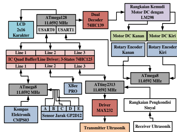
Gambar 3.2 Blok diagram Perangak Keras
