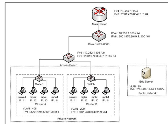
Gambar 2. Topologi EEPIS Net dengan Grid IPv6
